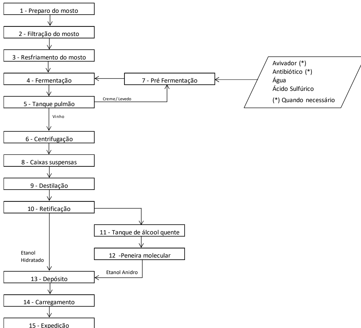
Fluxograma de fabricação - Etanol
